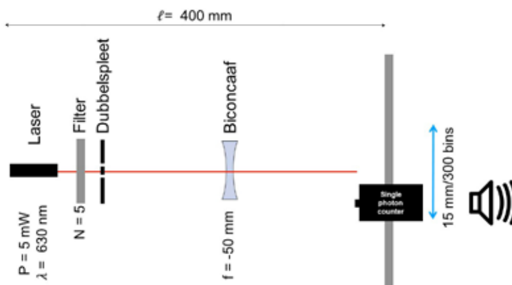
Figuur 1. Schema van het experiment
