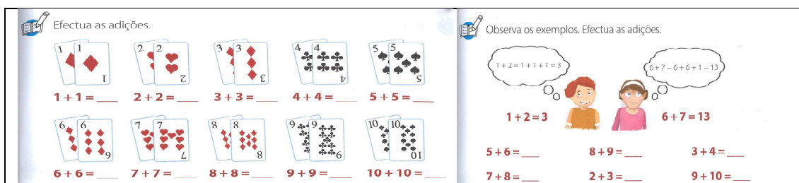
Fig. 7 The example elicits addition by the solution method of “doubles” or “doubles plus 1” in one of the Portuguese textbooks (Segredos dos Números 1, Matemática 1º ano o Ensino Básico, 2010, p. 99)
